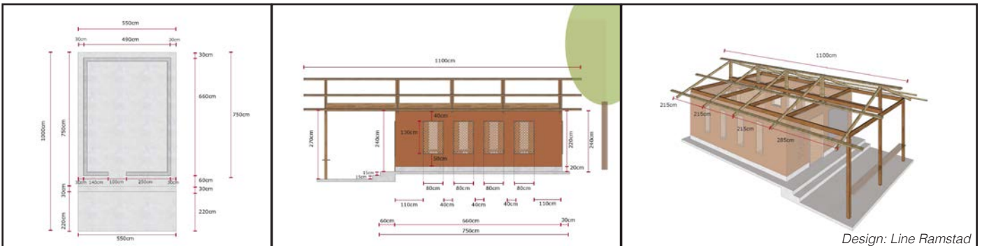
Arbeidstegninger for kontor og oppholdsareal for lærerne
